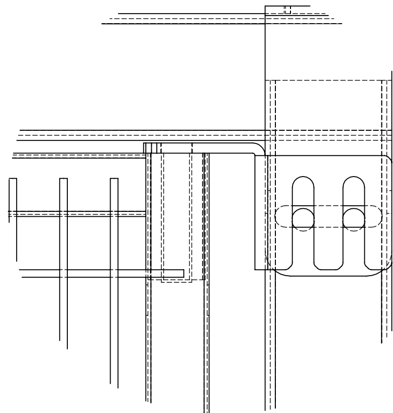
DETAY A ÖLÇEK 2:3
